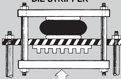
DIE STRIPPER
