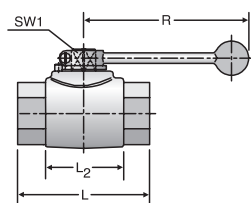
DN32-DN40
